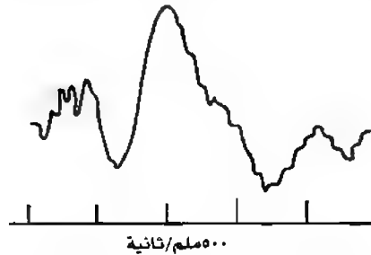
الشكل (٢ - ٩) فرق الجهد الكهربائي نتيجة استئارة ما
